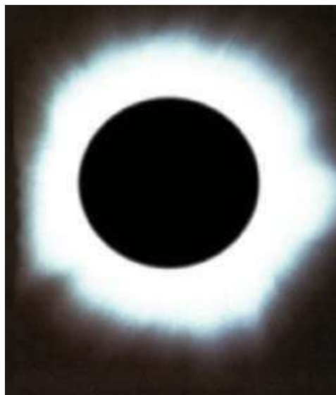
► Saulės užtemimas įrodo, kad Visata skendi tamsoje.
