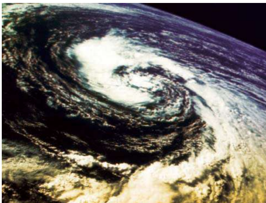
► Fotografijoje užfiksuoti atmosferoje esantys debesis bei vėjų srovės.
