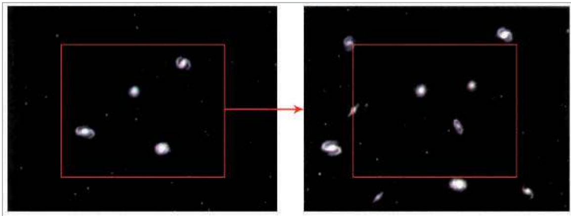
► Ši iliustracija demonstruoja didėjančius atstumus tarp galaktikų ar jų klasterių – Visata plečiasi.
